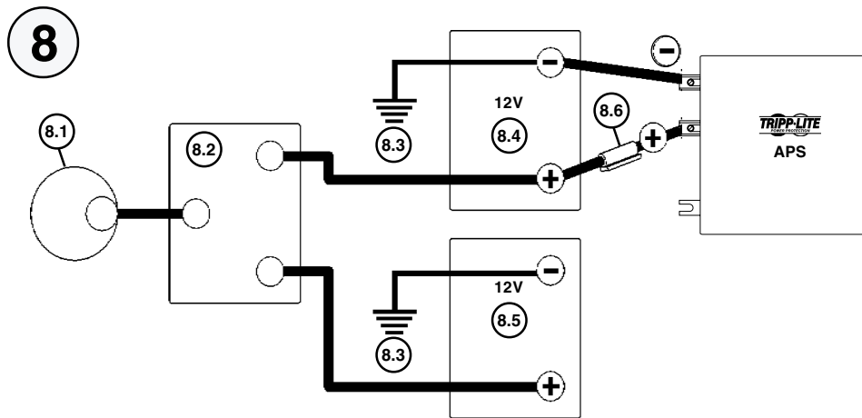
Advanced 12VDC Vehicular Battery Connection. See Pg.8. 8.1 is the alternator. 8.2 is a battery isolator. 8.3 is the vehicle battery ground. 8.4 is an auxiliary vehicle battery. 8.5 is the vehicle battery. 8.6 is the fuse. Conexión Avanzada de Baterías de 12V de CD en Vehículos. Vea página 24. 8.1 representa el alternador. 8.2 representa el aislador de la batería. 8.3 representa la conexión a tierra de la batería. 8.4 representa una batería auxiliar del vehículo. 8.5 representa la batería del vehículo. 8.6 representa el fusible.
